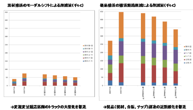
(図2 素材輸送のモーダルシフトと製品輸送の距離縮小による炭素排出削減量)
