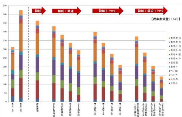
(図1 モーダルシフトによる輸送課程炭素排出量の変化)
